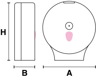
MAXI JUMBO PRESTIGE
